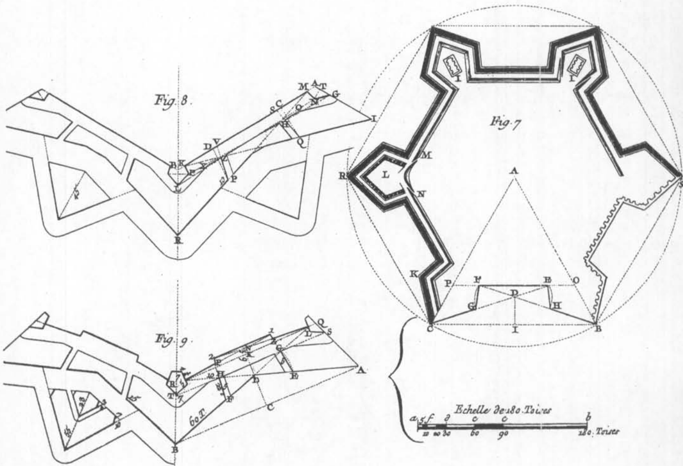
Fig. 7 : Het eerste verdedigingssysteem van Vauban. De streepjes lijnen en letters zijn constructielijnen. I zijn poedermagazijnen op ieder uitzichtpunt. M en N zijn hellende toegangen voor manschappen en kanonnen naar ieder bastion.
